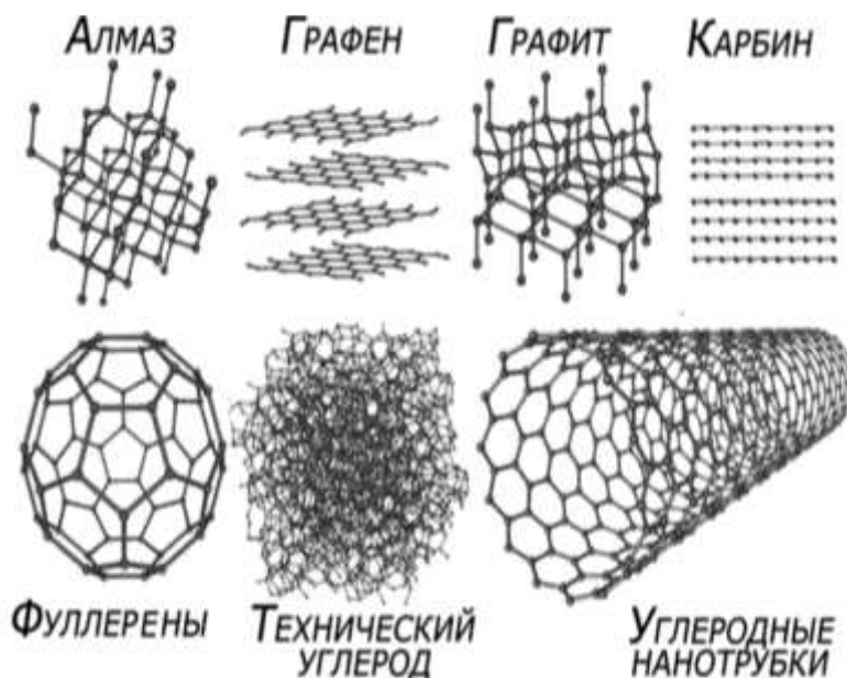
Рисунок 5 – Структура нанотрубок
