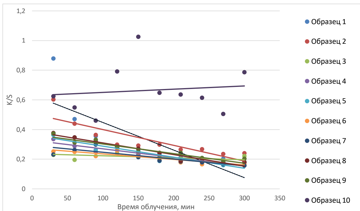
Рис. 4. Эффективность фотокаталитического разложения МГ титансодержащими золями
